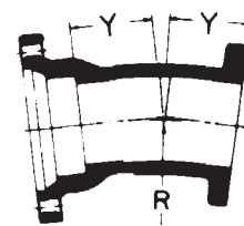
11 1/4° MJxFLG (1/32)
