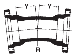
11 1/4° MJ (1/32)
